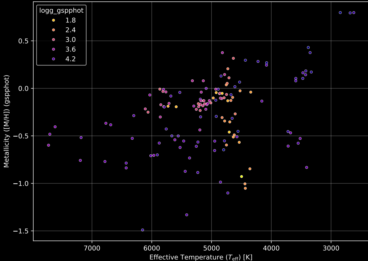
APOGEE DR17 Field: [349+22-O] Stellar Population Parameters (n= 143)
